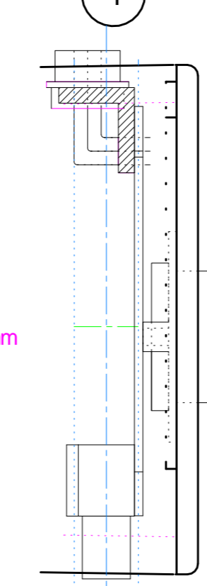
Aufsicht Deckel 4 Deckel aufgesetzt
