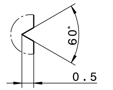
Detail A 10:1
