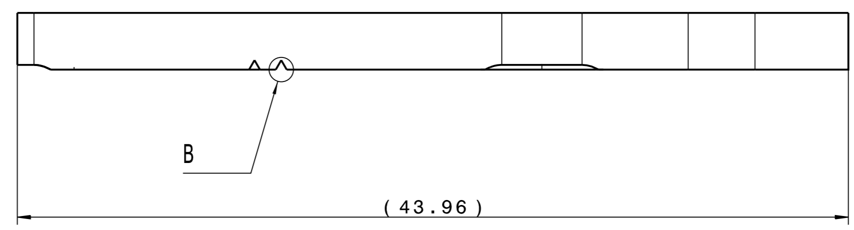
Detail B 10:1
