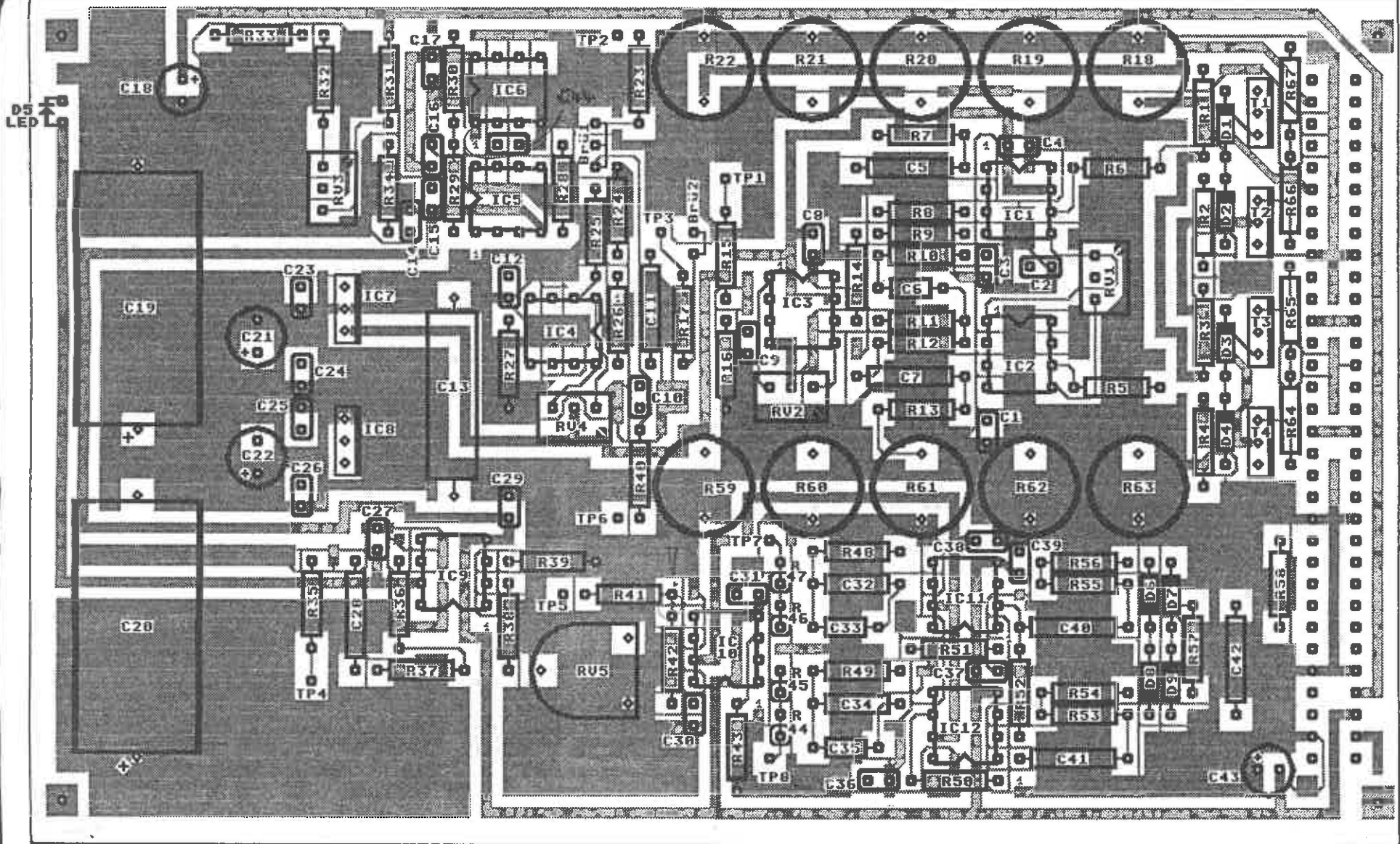
GSI REGELVERSTÄRKER FG 376 850 Bestückungsplan und Steckerbelegung
